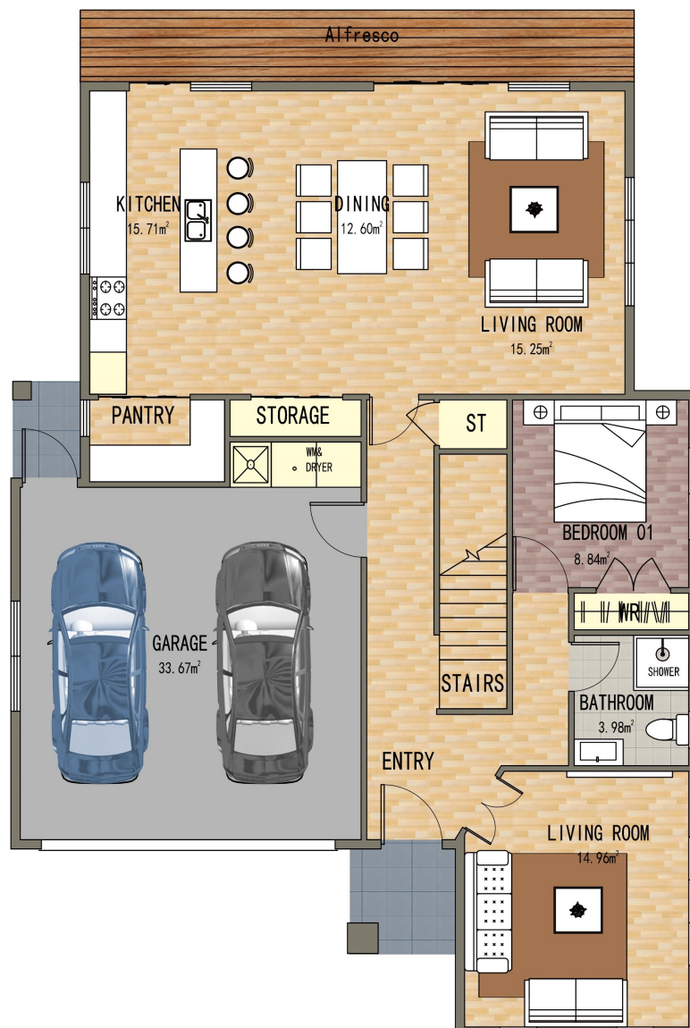
一层户型图
